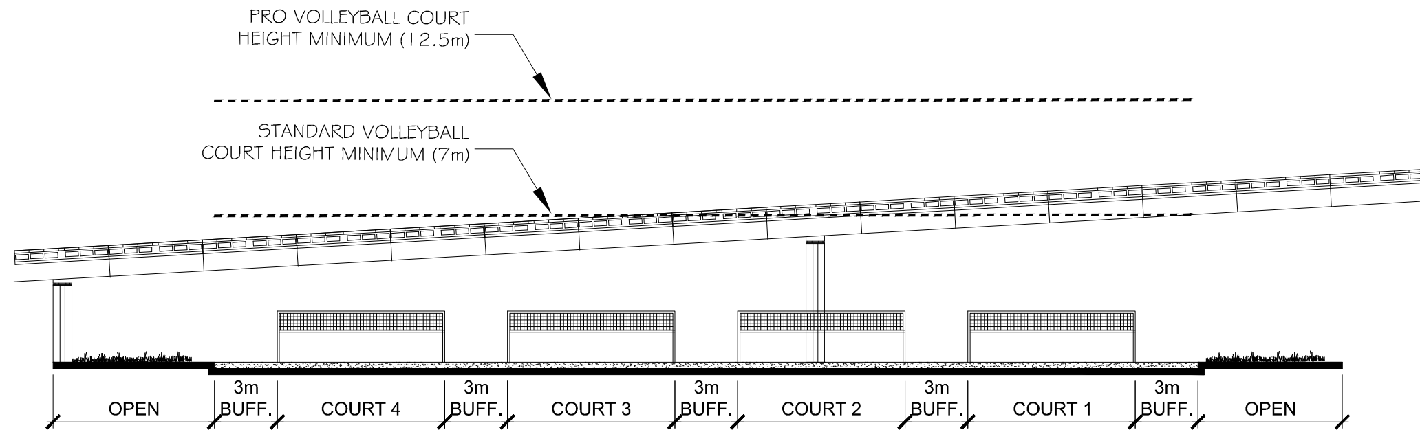
ELEVATION C-C
