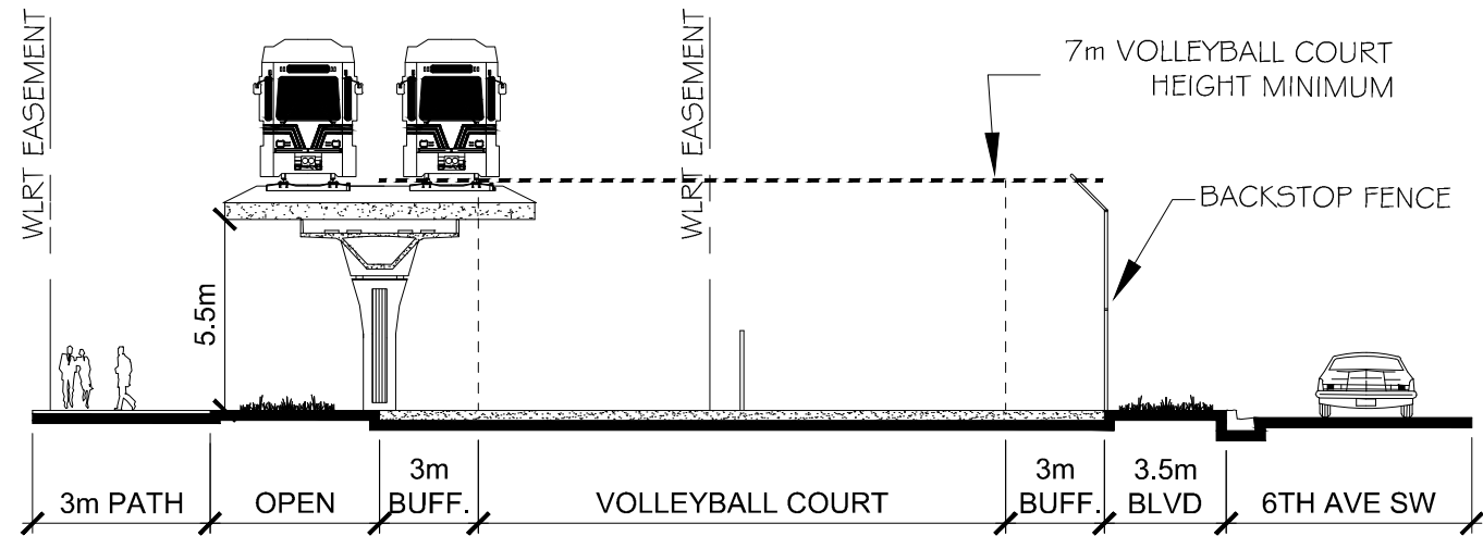
ELEVATION B-B
