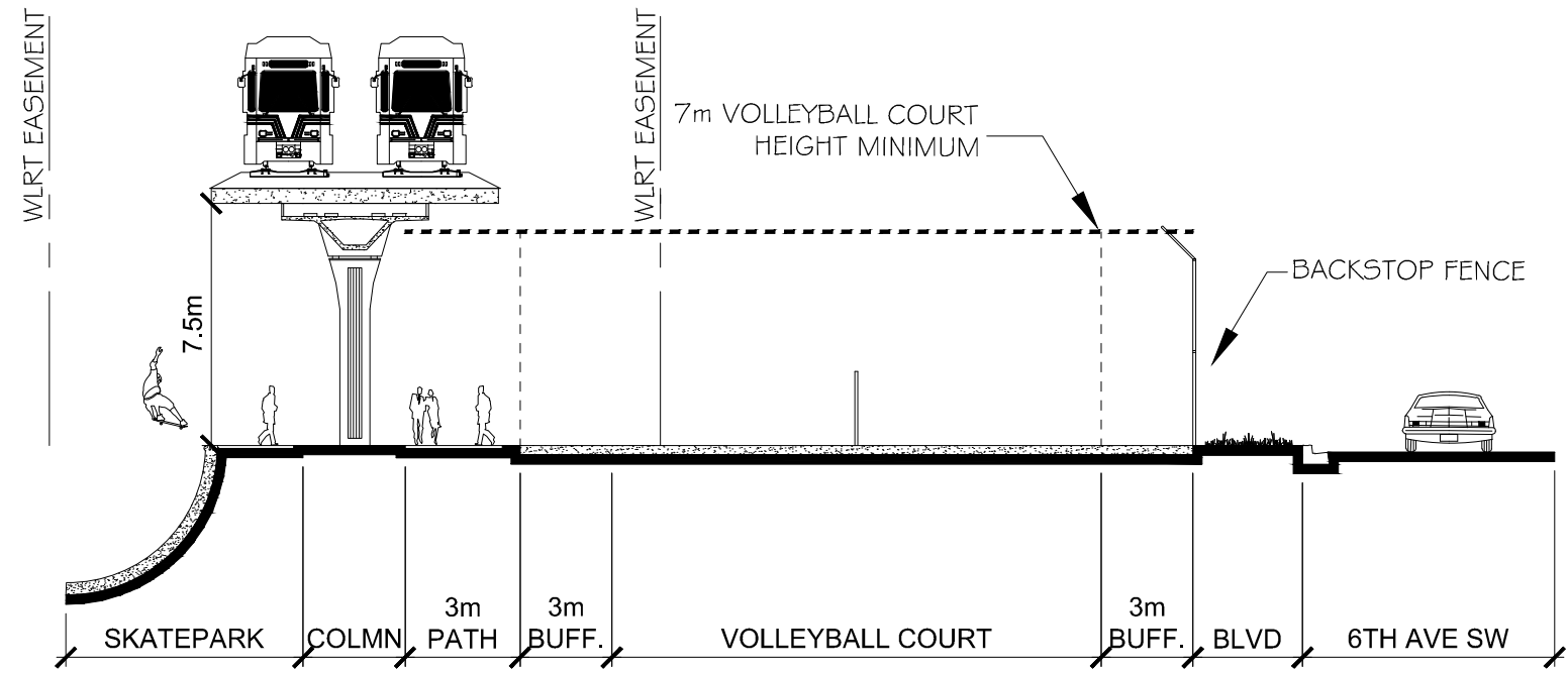
ELEVATION A-A
